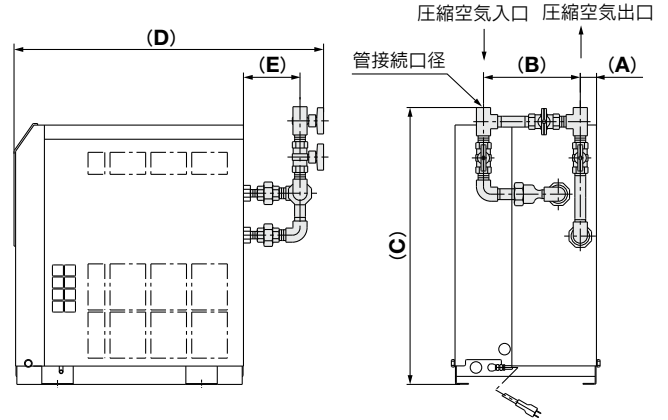
寸法表 (mm)
