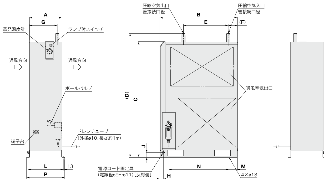
寸法表
