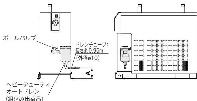
寸法表 (mm)
