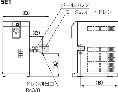
寸法表 (mm)
