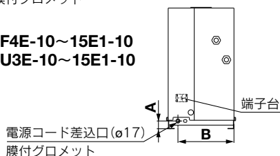
寸法表 (mm)
