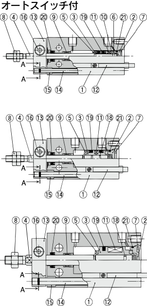
構成部品
